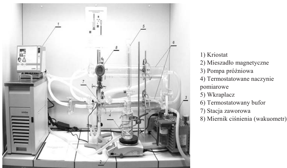
Rys. 4. Instalacja laboratoryjna do badań procesów absorpcji CO 2
